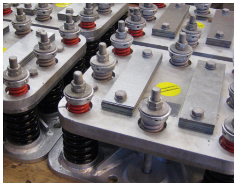
TMD in production 生产中的调谐质量阻尼器
