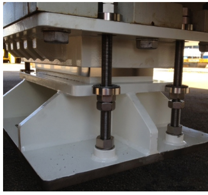
Cushion Anti-Vibration Mount 重型垫式式减振底座
